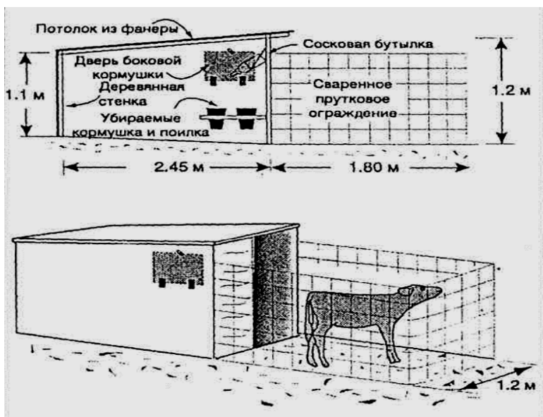
Рисунок 22 – Индивидуальное размещение телят в деревянныхдомиках
