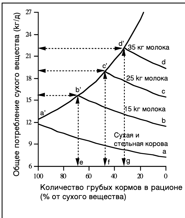
Рисунок 4: Влияние производства молока (энергетическая потребность) на оптимальное процентное содержание грубых кормов в рационе, максимально увеличивающее их использование и позволяющее корове полностью проявить ее генетический потенциал производства молока.
