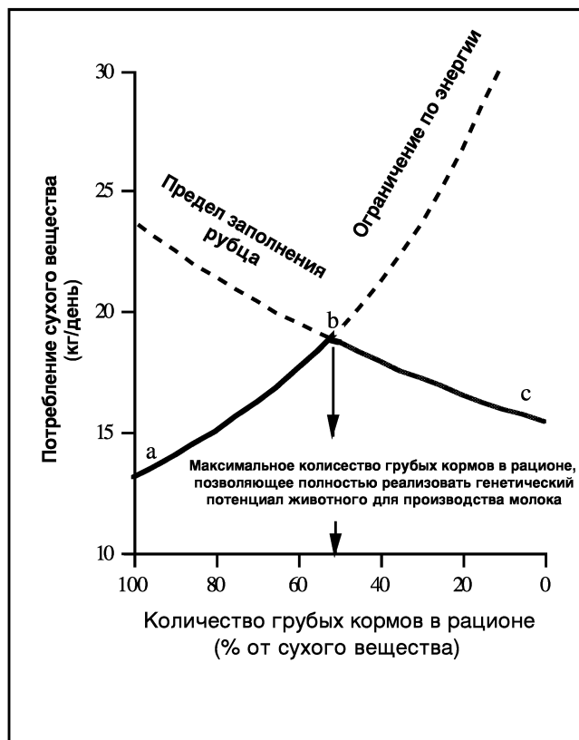
Рисунок 3: Влияние соотношения грубых кормов и концентратов на потребление сухого вещества рациона. Если рацион коровы содержит большое количество грубых кормов (фуража), то наполнение желудка ограничивает потребление кормов. Добавление в рацион концентратов увеличивает потребление общего количества кормов (линия от А до Б). С другой стороны, если рацион коровы состоит из диеты с низким содержанием грубых кормов (высоким содержанием концентратов), насыщение организма энергией регулирует потребление кормов. В этом случае добавление в рацион концентратов уменьшает потребление общего количества кормов (линия от Б до С), так как энергетические потребности организма животного могут быть удовлетворены при потреблении значительно меньшего количества кормов.
