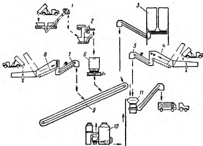
Рис. 12. Технологическая схема комплекта оборудования кормоцеха КОРК-15:
