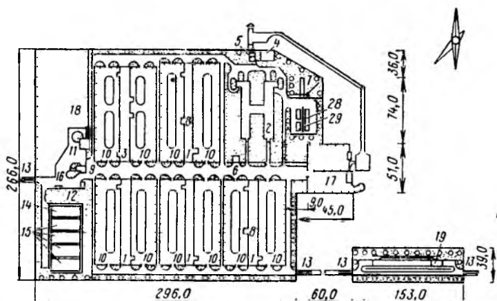
Рис. 19. Ферма мясного скота на 800 голов:
