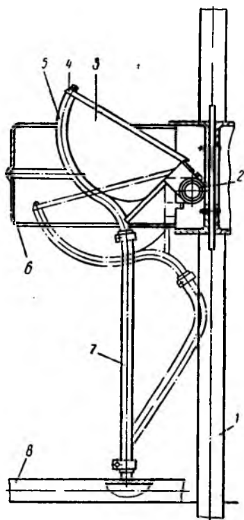
Рис. 16. Установка поильной чаши автопоилки групповой поплавковой АГП-Ф-200
