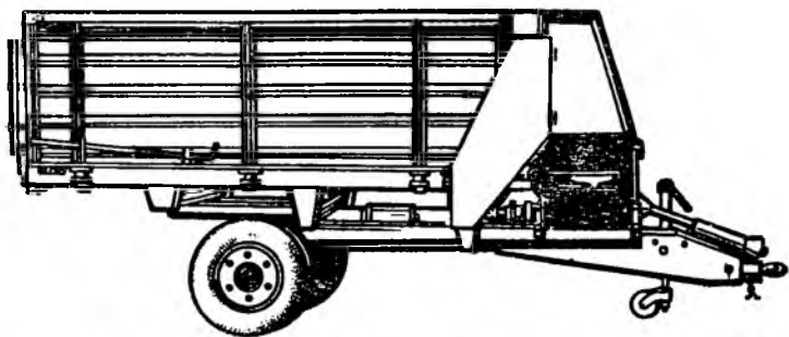
Рис. 13. Раздатчик кормов мобильный малогабаритный РММ-Φ-6
