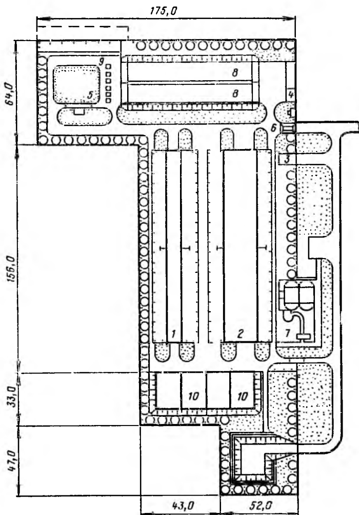
Рис. 18. Площадка для откорма молодняка на 1 тыс. ското-мест:
