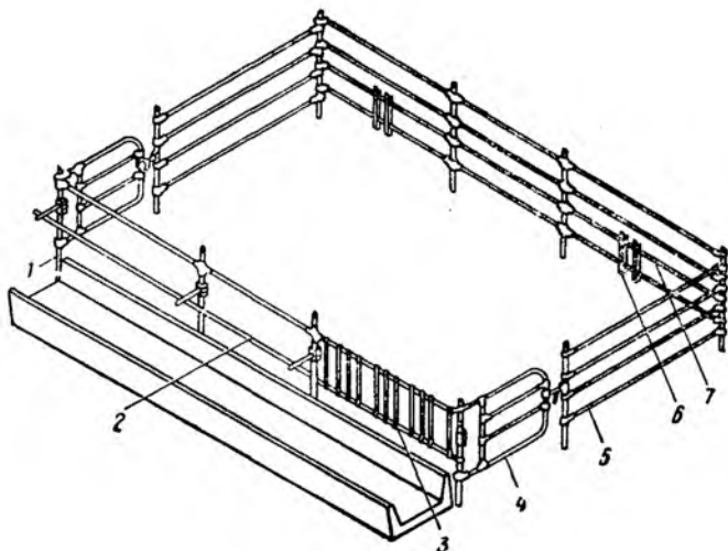
Рис. 11. Клетка групповая из унифицированных элементов для молодняка крупного рогатого скота:
