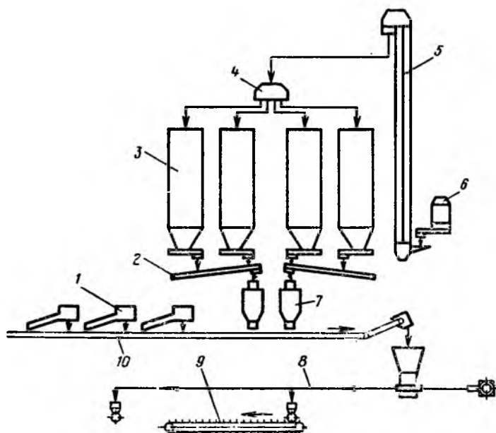
Рис. 15. Поточная линия приготовления и раздачи кормов молодняку крупного рогатого скота из модернизированного комплекта машин и оборудования КПГ-10А:
