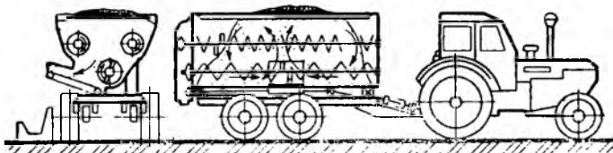
Рис. 14. Раздатчик-смеситель кормов прицепной РСП-10
