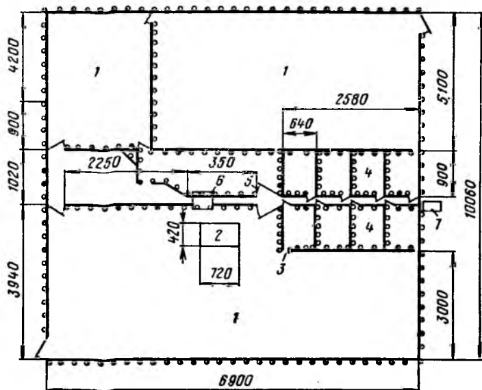
Рис. 3. Площадка для осмотра и сортировки скота:
